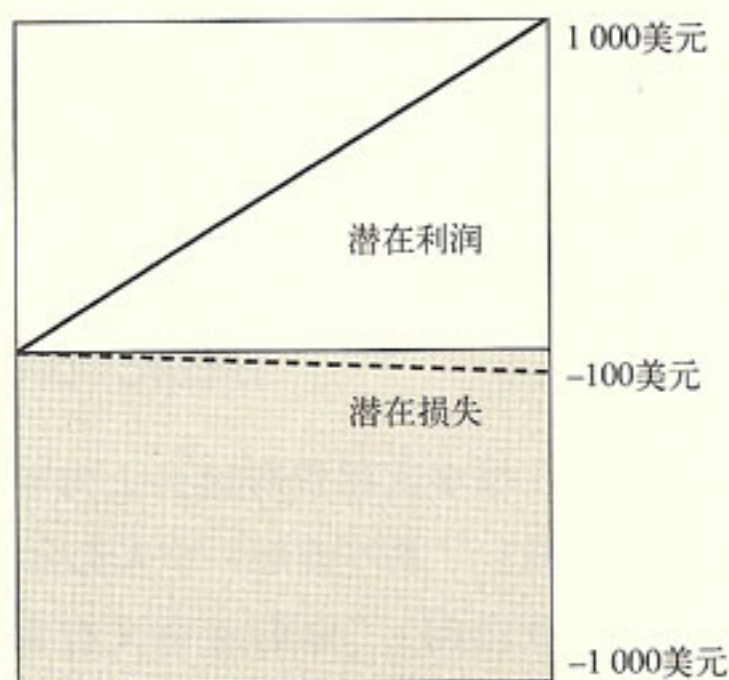
图3-2 高概率事件
